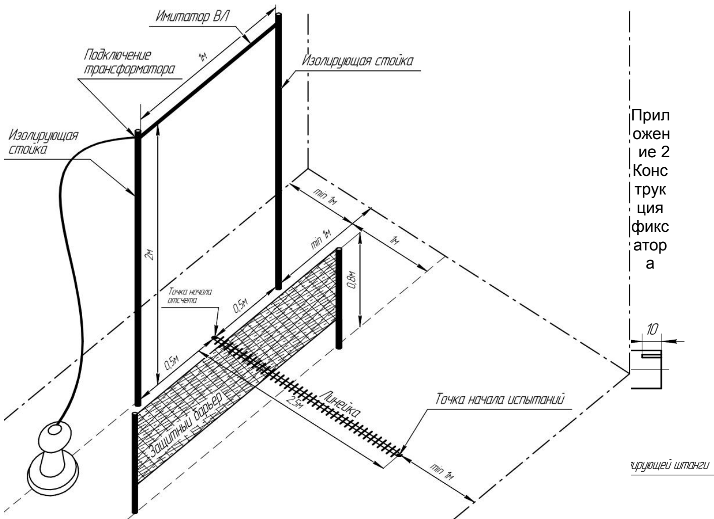
Стенд для проверки чувствительности СНК «Купол»
